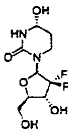
Composé 1a.
