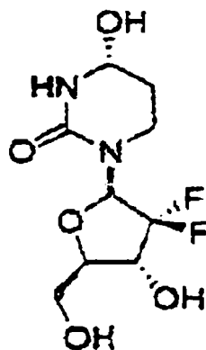
Verbindung 1a.
