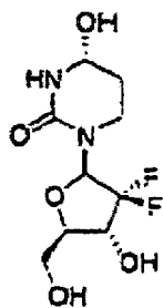
Composé 1a.
