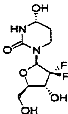
Verbindung 1a.
