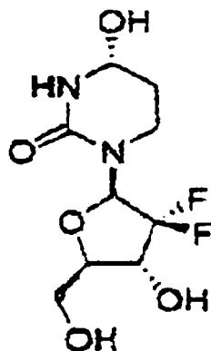
Verbindung 1a.
