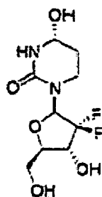
Composé 1a.
