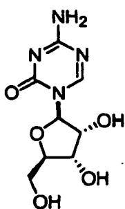
5-azacytidine
