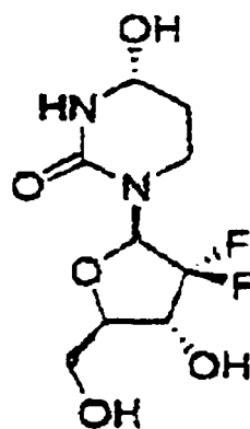
Verbindung 1a.
