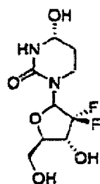
Composé 1a.
