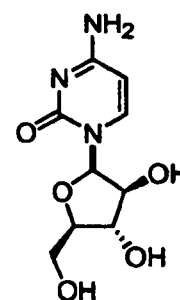
ara-C
