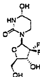
Composé 1a.
