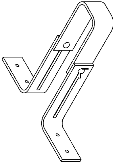
FIG. 9A. ISOMETRIC NOT TO SCALE
