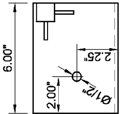
FIG. 12C. SIDE
