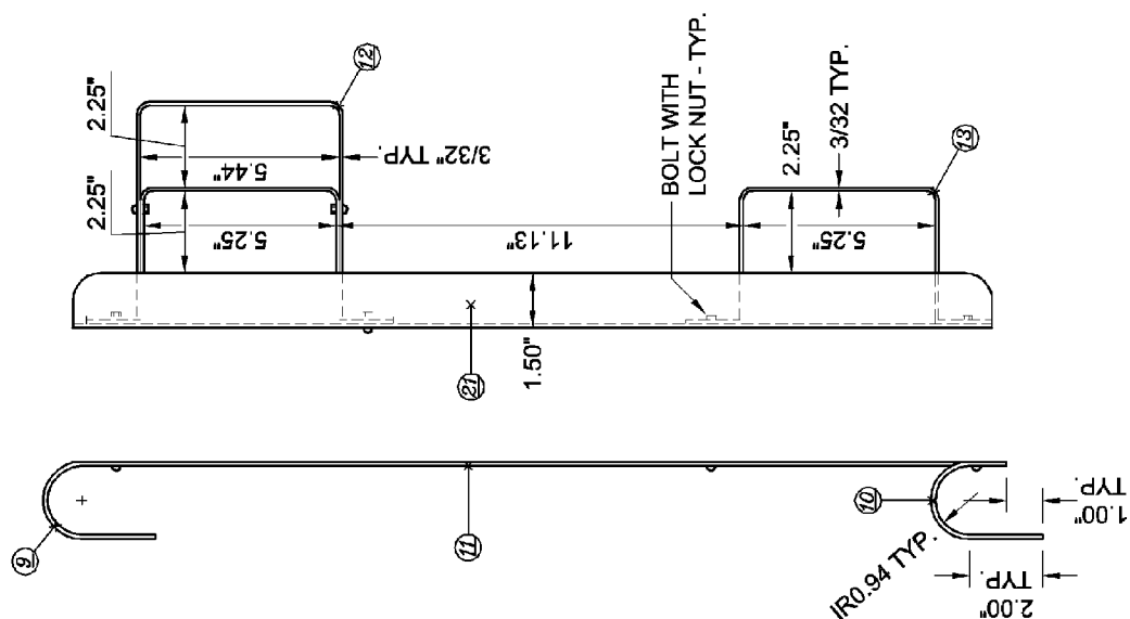
FIG. 21C. SIDE
