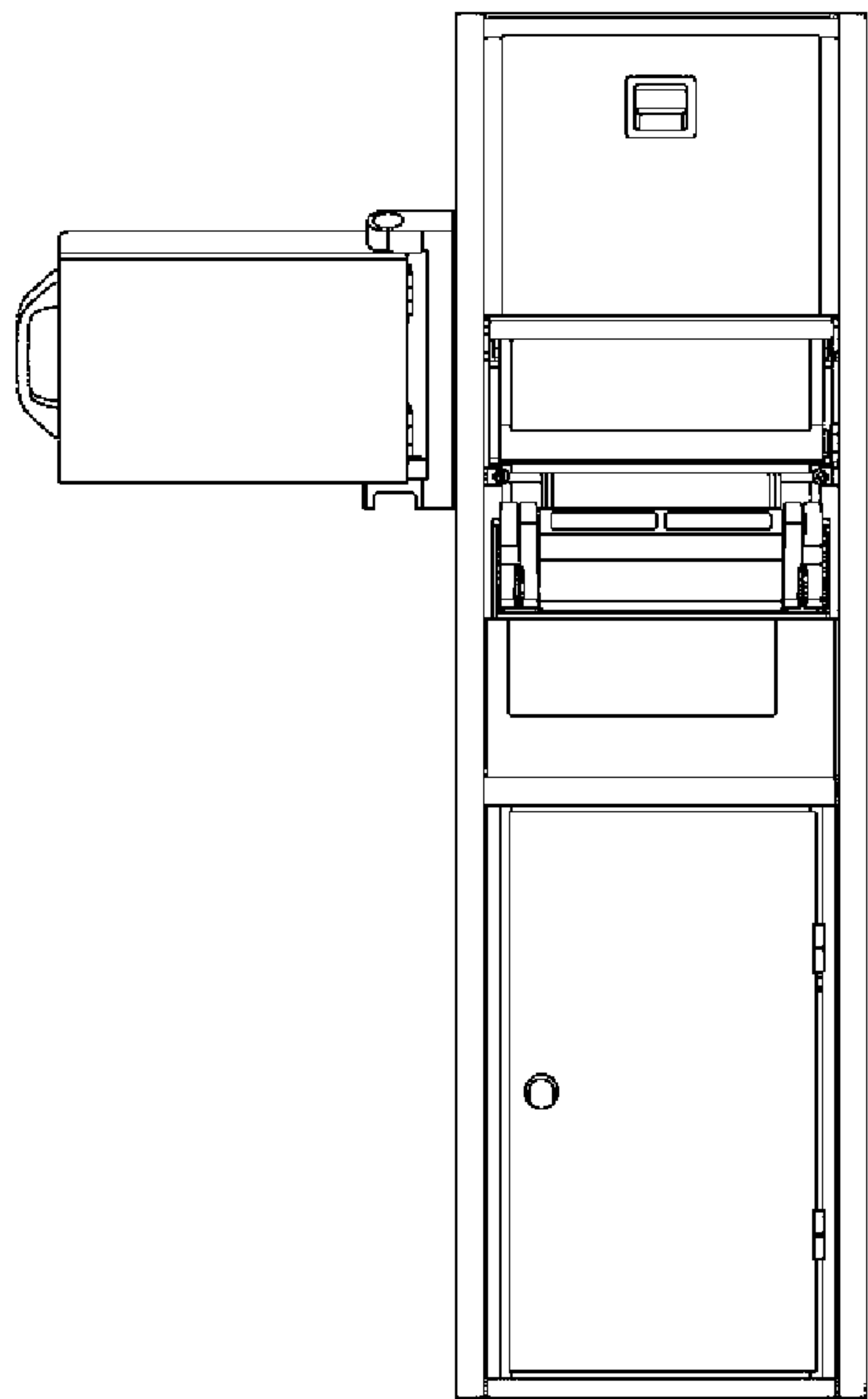
【後視圖】
