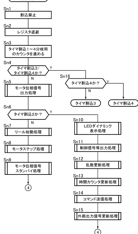
【図 41】 タイマ割込処理(メイン)
