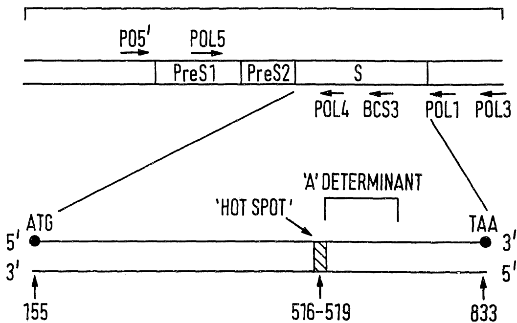
FIG. 3 P ORF
