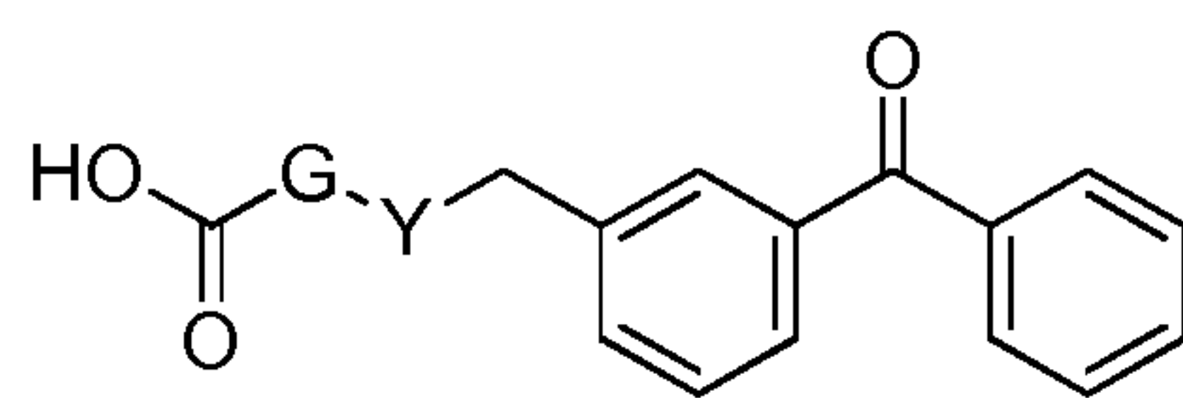
(IV)
