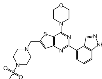
GDC-0941
