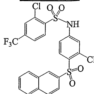
2-Chloro-N-[3-chloro-4-(naphthalene-2-sulfonyl)-phenyl]-4-trifluoromethylbenzenesulfonamide(105)
