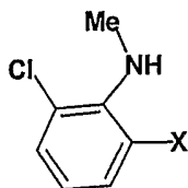
355 X=NO 2 356 X=NH 2
