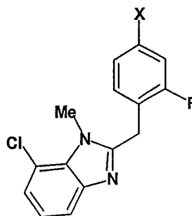
357 X=NO 2 358 X=NH 2
