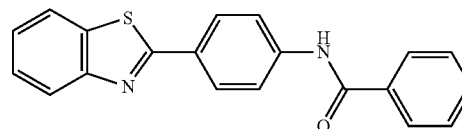
N-(4-Benzothiazol-2-yl-phenyl)-benzamide
