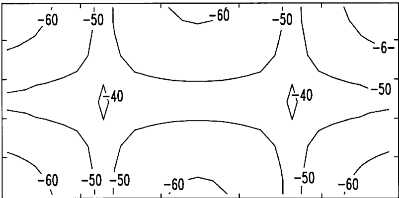
FIG. 6 BOUNDARY DIFFUSION
