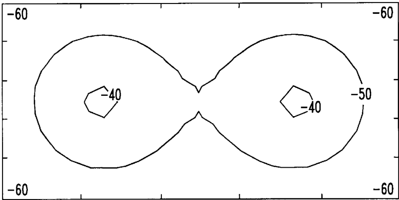
FIG. 5 BULK DIFFUSION
