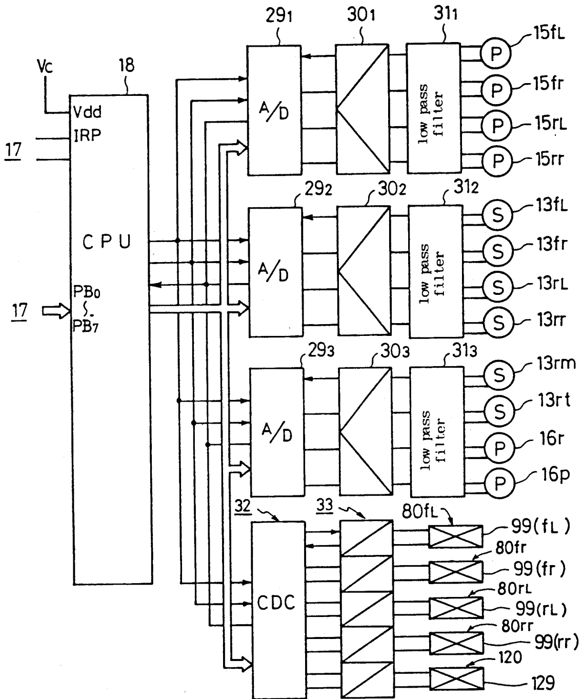
Fig. 8b
