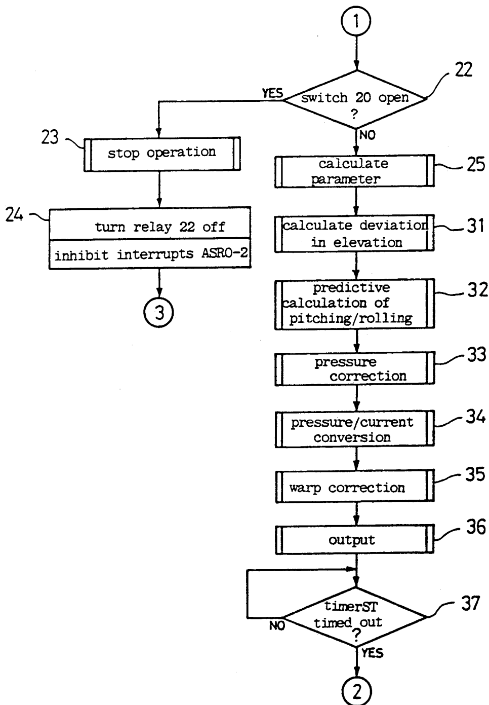
Fig. 9c
