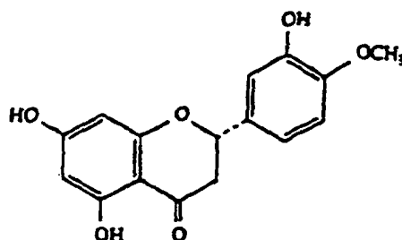
Hesperetin
