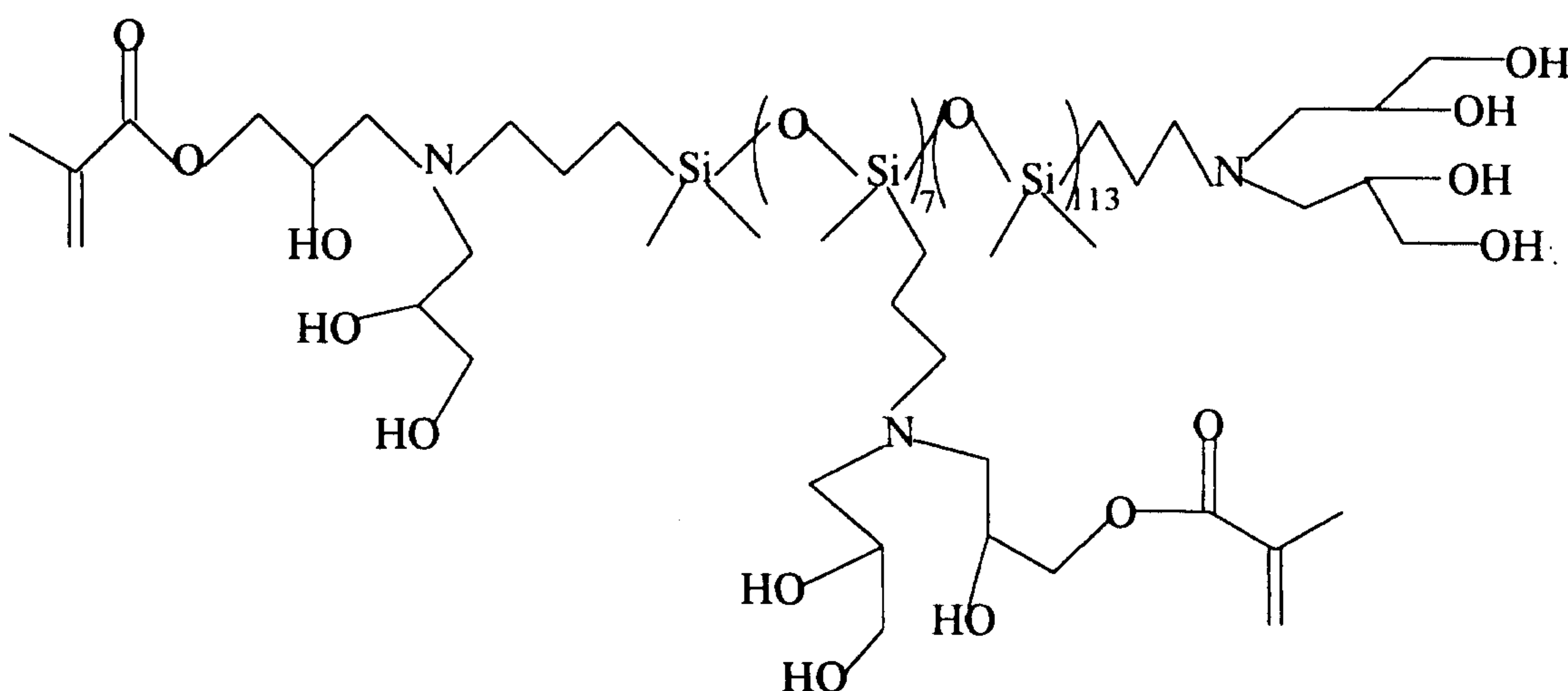
Structure XIV.
