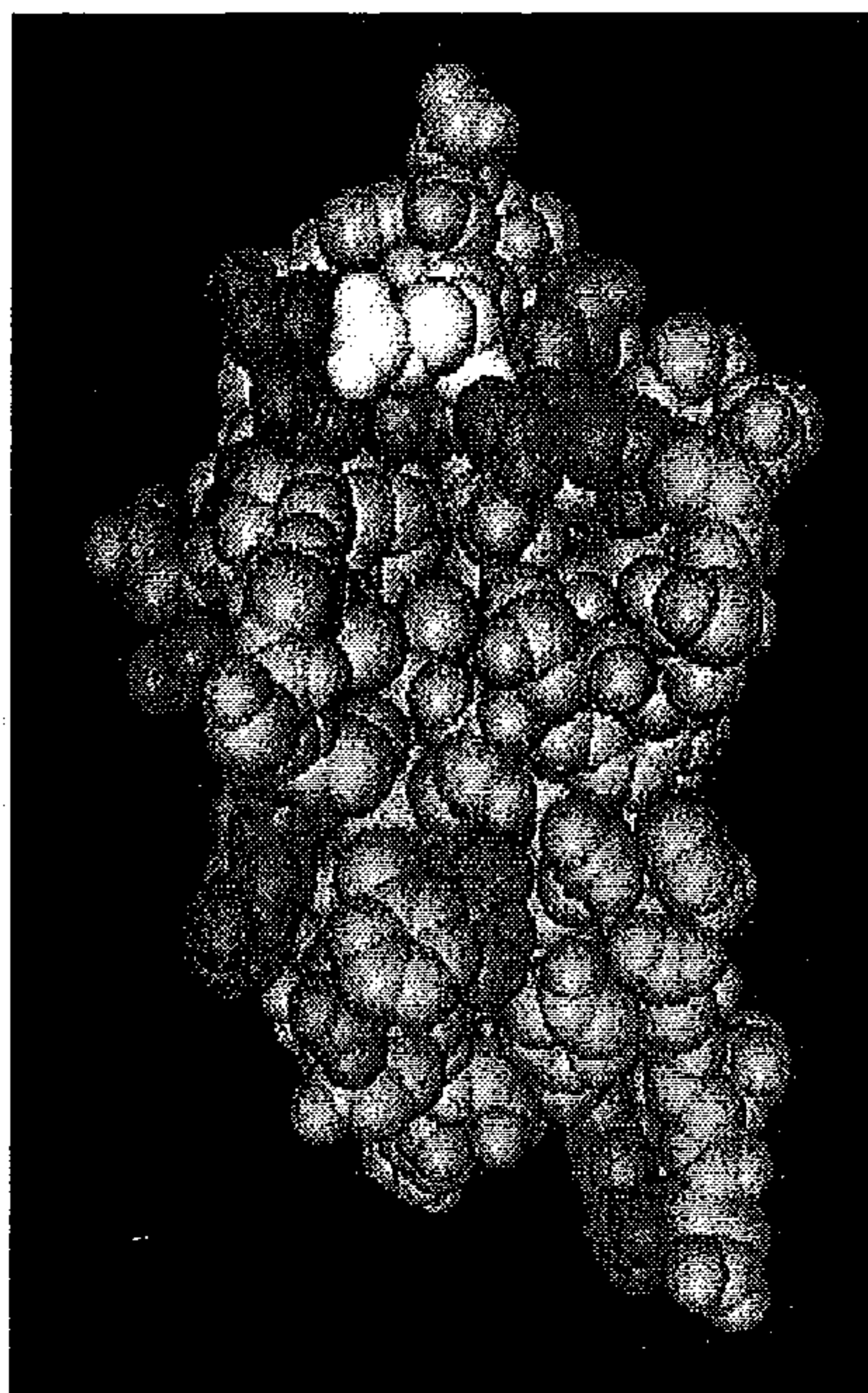
V λ 6 Wil Glu81
