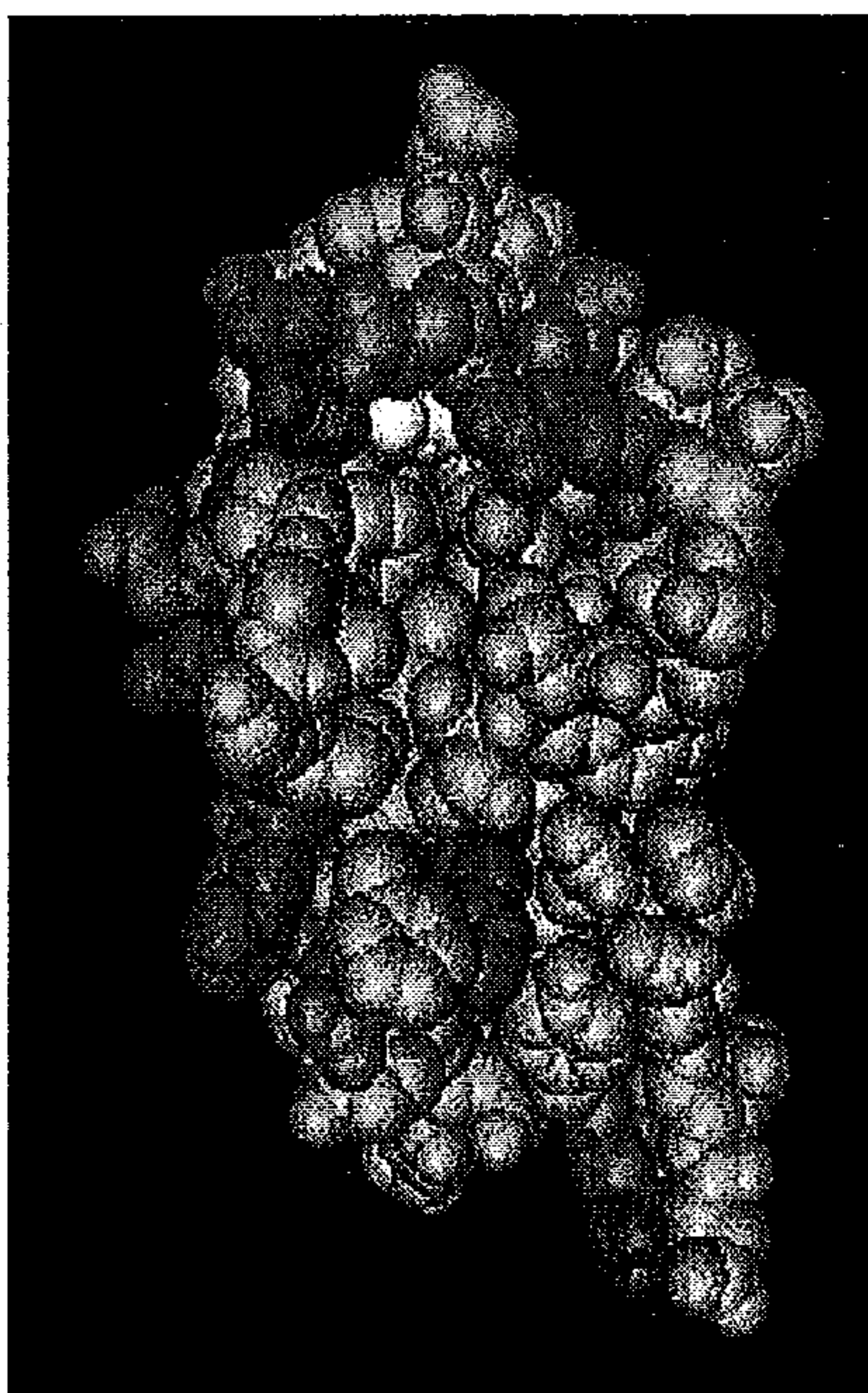
V λ 6 Wil Asp82
