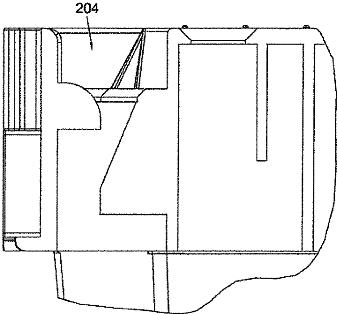
Fig. 74 SECTION D-D
