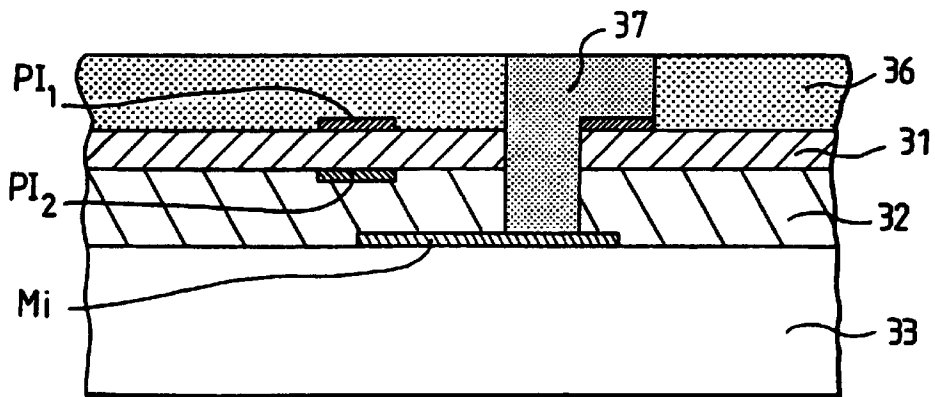
SECTION ON DD
