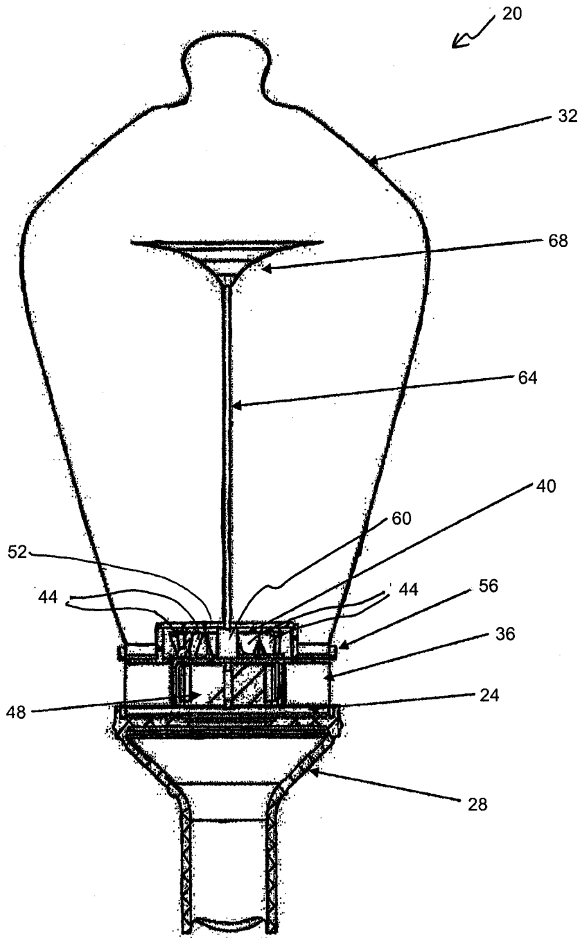
SECTION A-A
