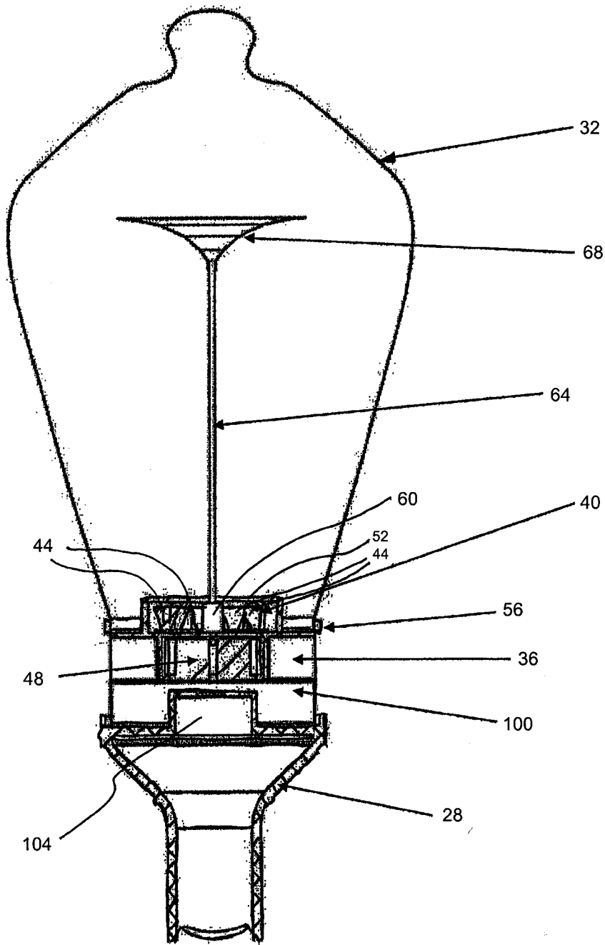
SECTION A-A
