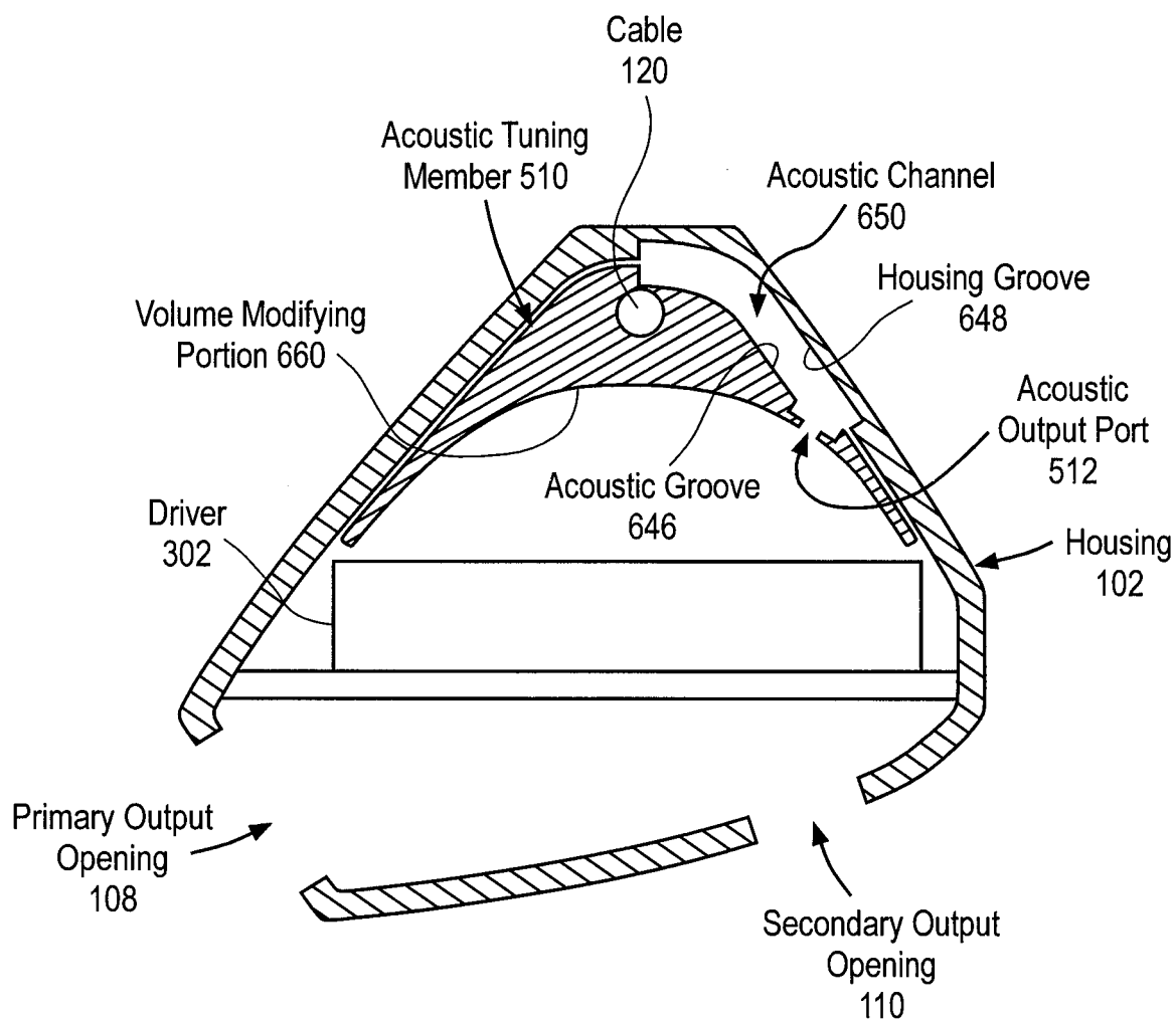
FIG. 6C
