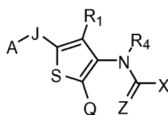
Formula (VI);
