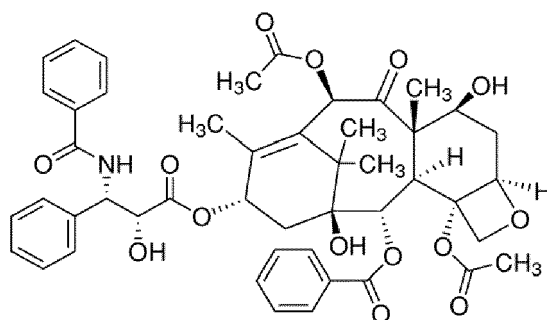
paclitaxel
