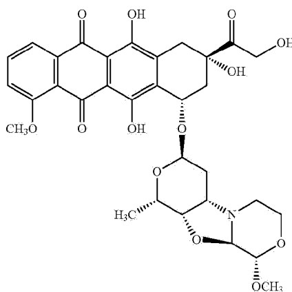
PNU-159682
