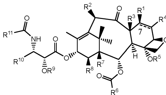
D-II,
