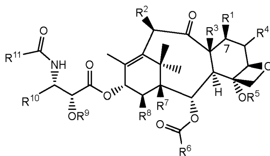
D-I,
