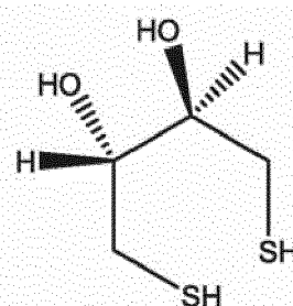
Dithiothreitol (DTT)
