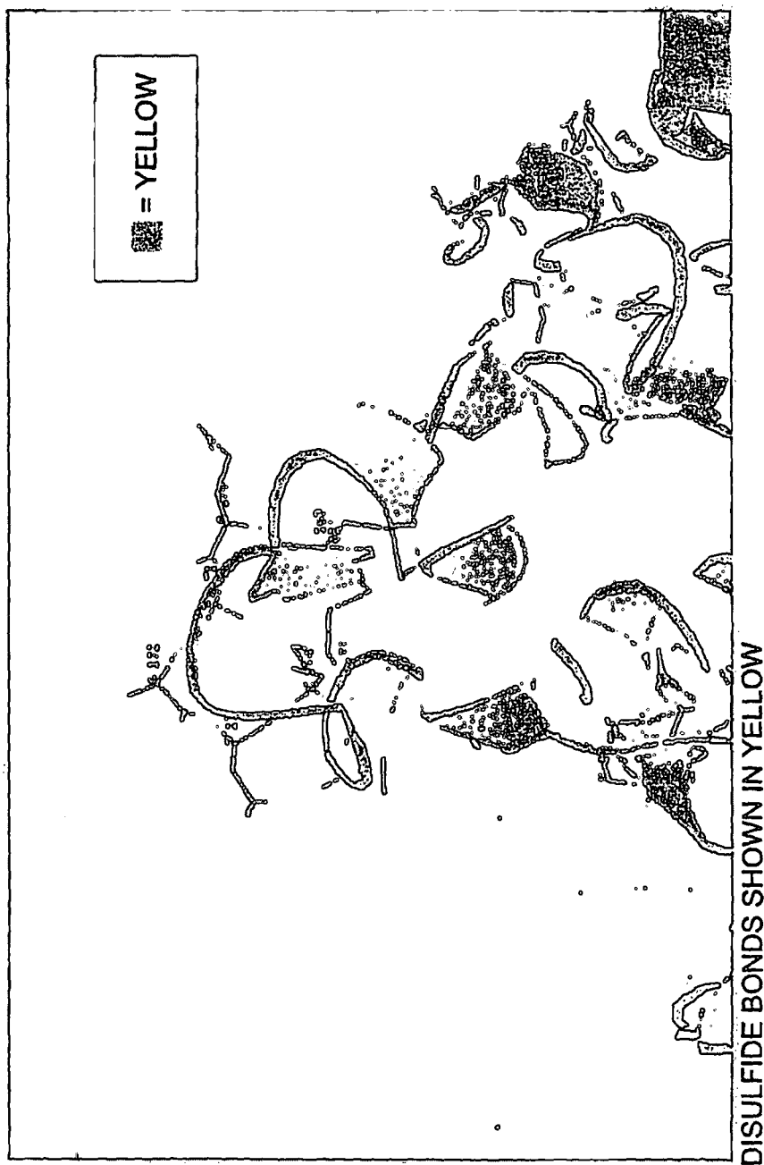
FIG. 12: LOOP IV GLU170-A176
