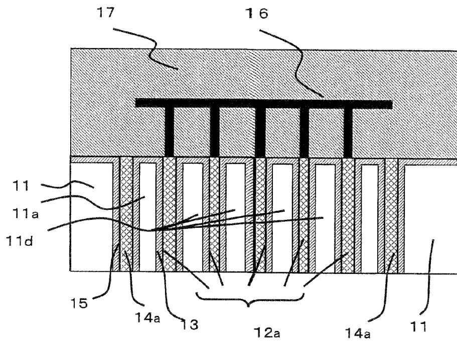
FIG. 10A
