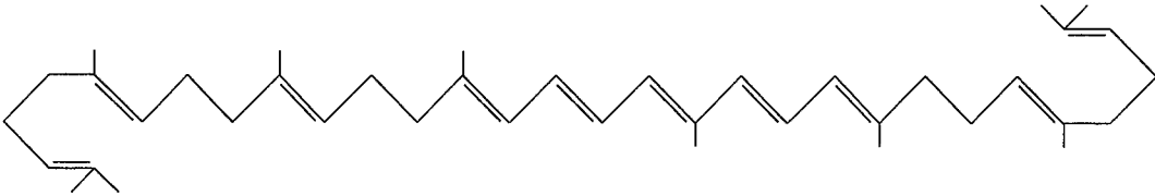
PHYTYLUENE
