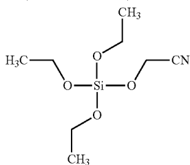
3-(Triethoxysilyl) propionitrile (CAS: 919-31-3)
