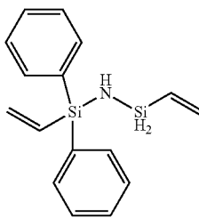
[ethenyl-(ethenylsilylamino)-phenylsilyl]benzene
