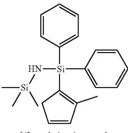
[(2-methylcyclopenta-1,3-dien-2-yl)-phenyl-(trimethylsilylamino)silyl]benzene
