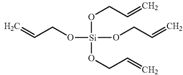
tetraallyl orthosilicate (CAS: 1067-43-2)
