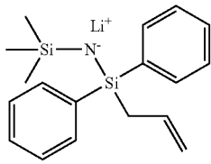
N-(Allyldiphenylsilyl)trimethylsilylaminolithium
