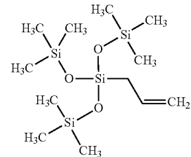
Allyltris(trimethylsiloxy)silane (CAS: 7087-21-0)
