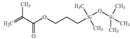
(3-Methacryloxypropyl)pentamethylsiloxane
