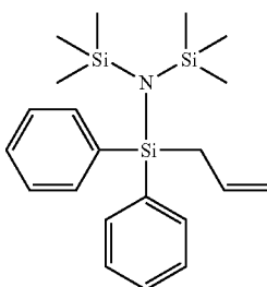
N-(Allyldiphenylsilyl)bis(trimethylsilyl)amine
