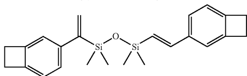
1-[(E)-2-(Bicyclo[4.2.0]octa-1,3,5-trien-3-yl)viny]-3-[1-(bicyclo[4.2.0]octa-1,3,5-trien-3-yl)viny]-1,1,3,3-tetramethyldisiloxane
