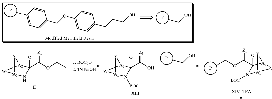
Scheme VI
