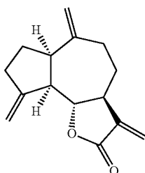
Dehydrocostuslactone
