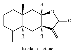
Isoalantolactone
