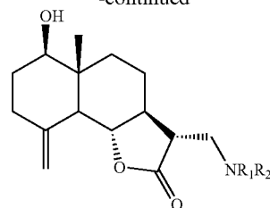
(+)-Aminoreynosin
