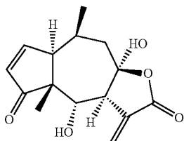
Helenalin
