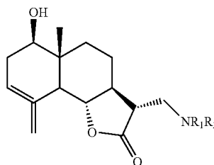
Aminosantamarins
