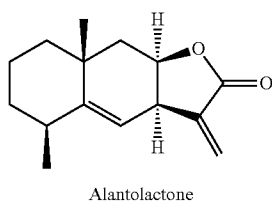
Alantolactone
