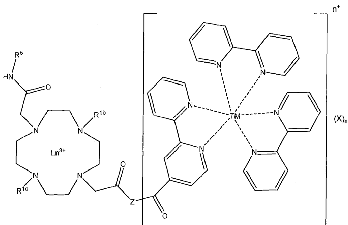
Formule B
