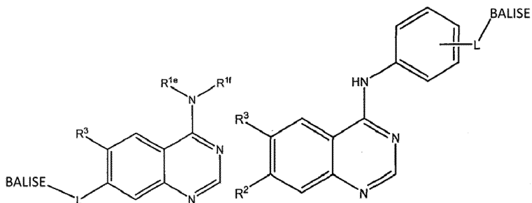
Formule III
