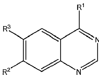
Formule I
