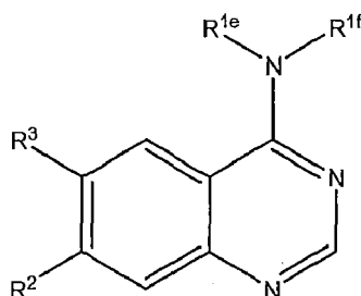
Formule II
