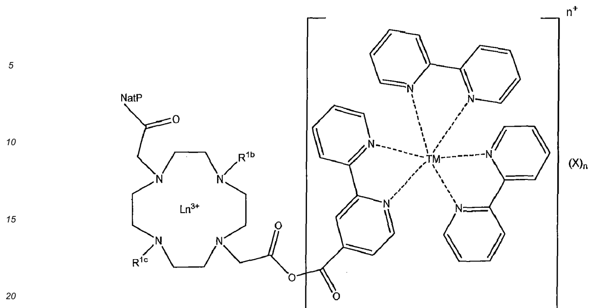
Formule H
