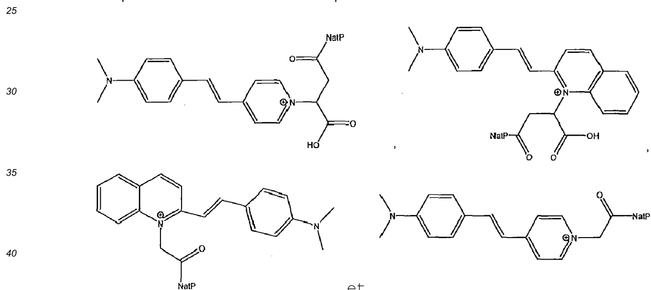
Formule H
