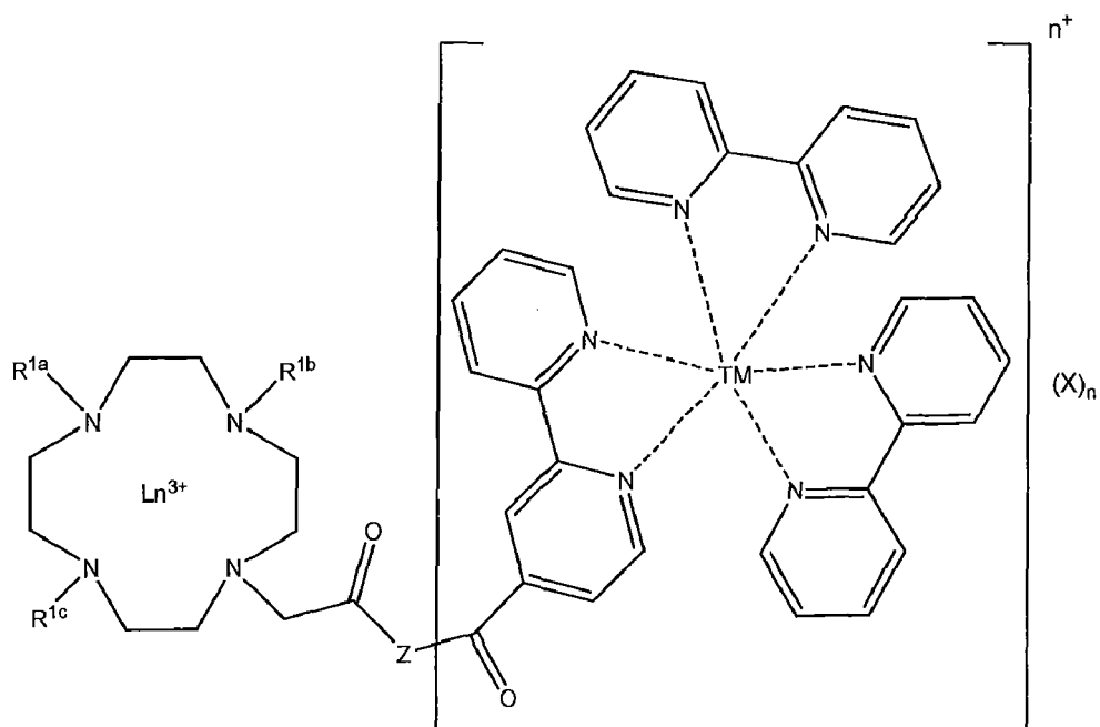
Formule A
