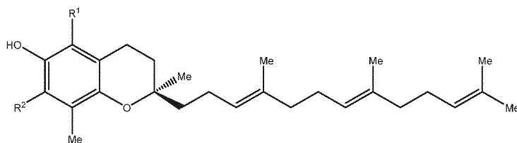
Tocotrienol
