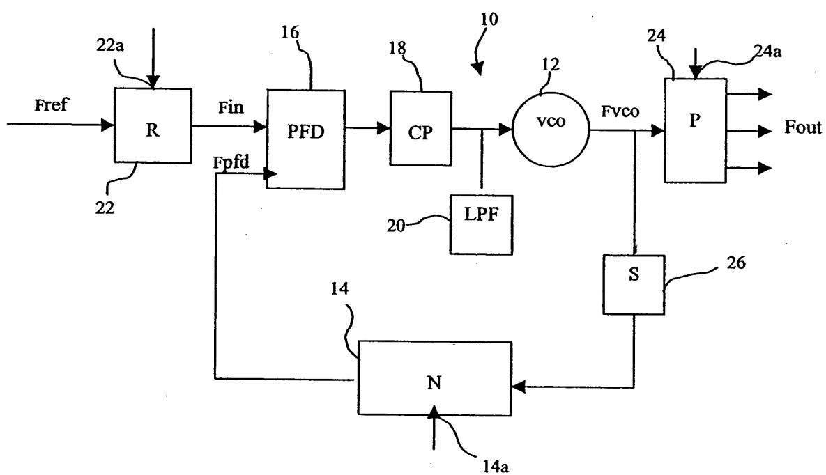
FIG. 1 (art antérieur)
