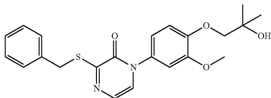
3-(benzylthio)-1-(4-(2-hydroxy-2-methylpropoxy)-3-methoxyphenyl)pyrazin-2(1H)-one
