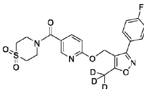
Formule II.
