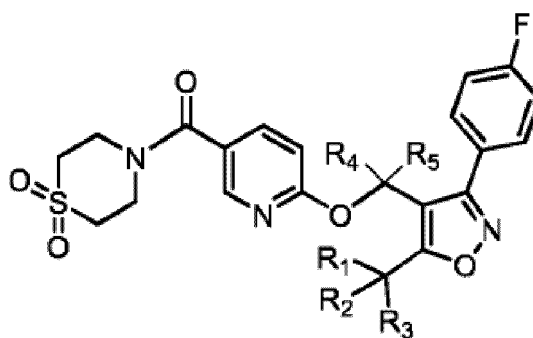
Formule I
