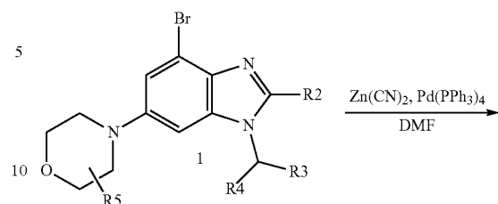
Scheme VI
