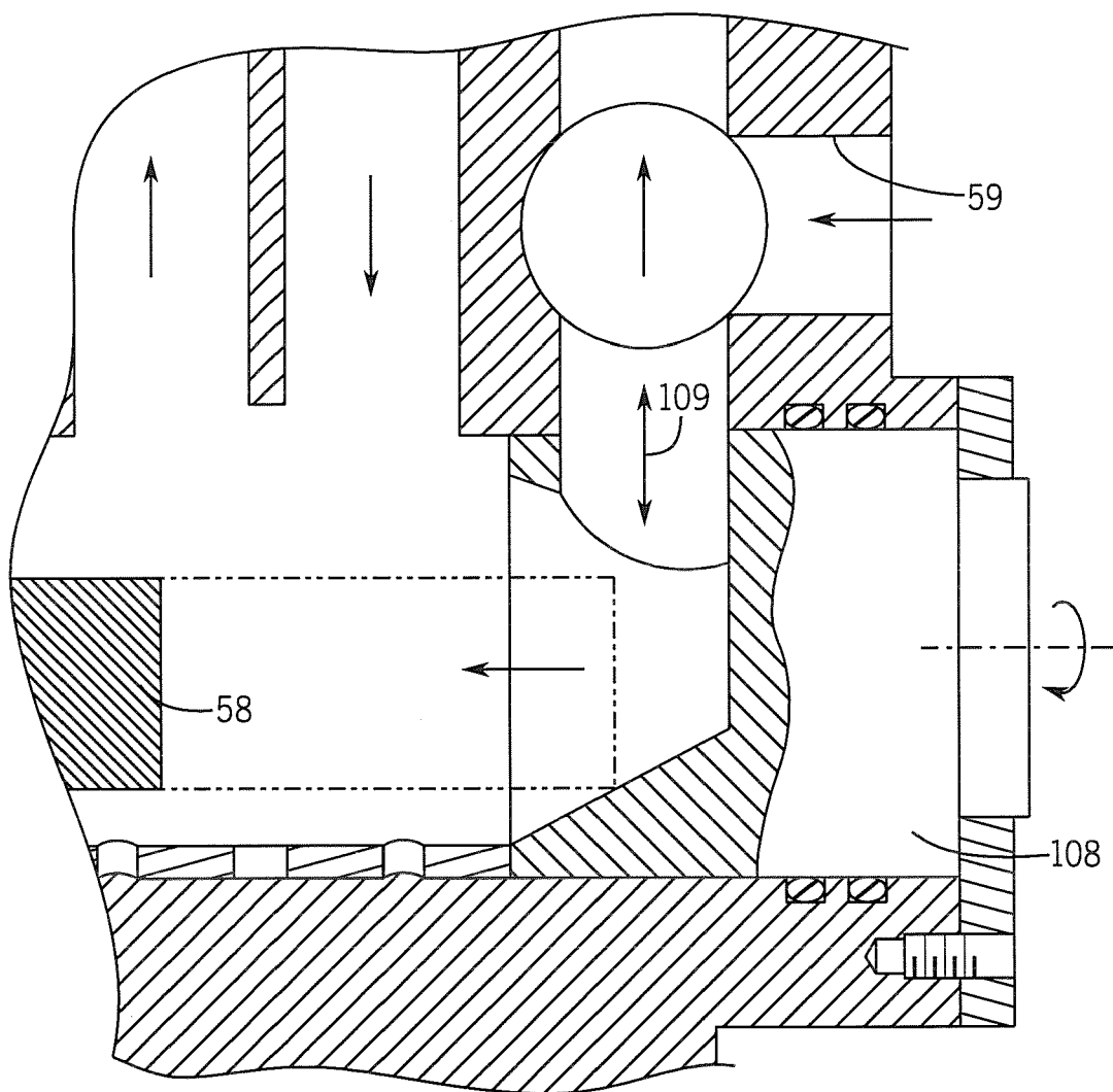
FIG. 12B
