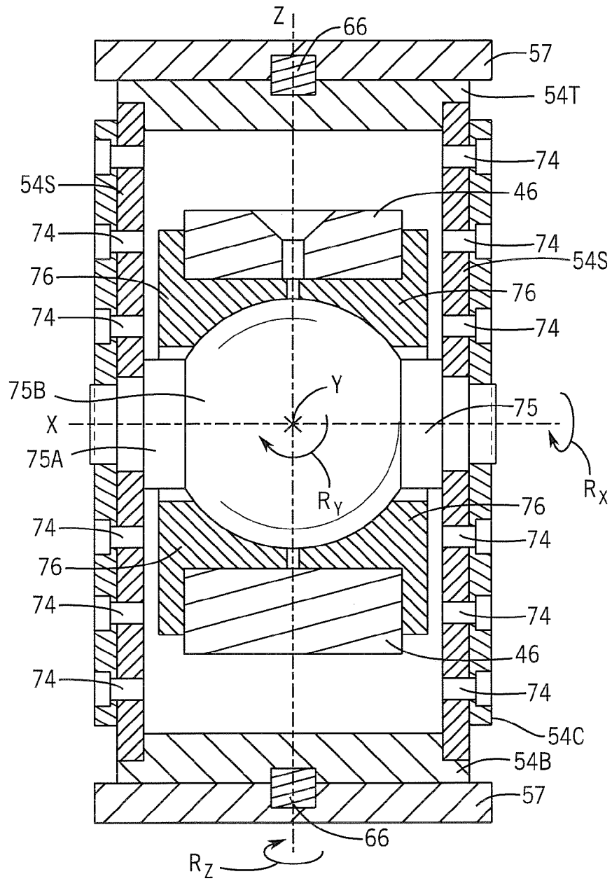
FIG. 8A
