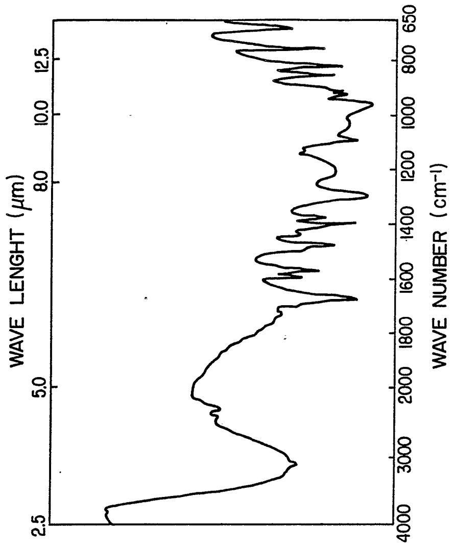
FIG. 2 IR SPECTRUM
