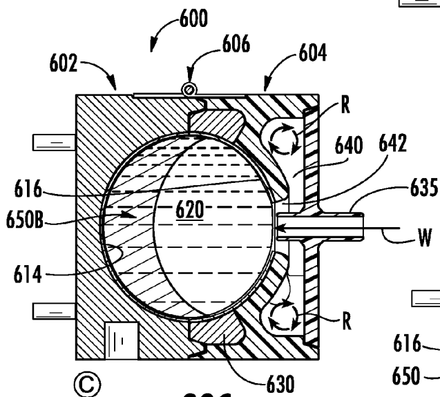
FIG. 33C
