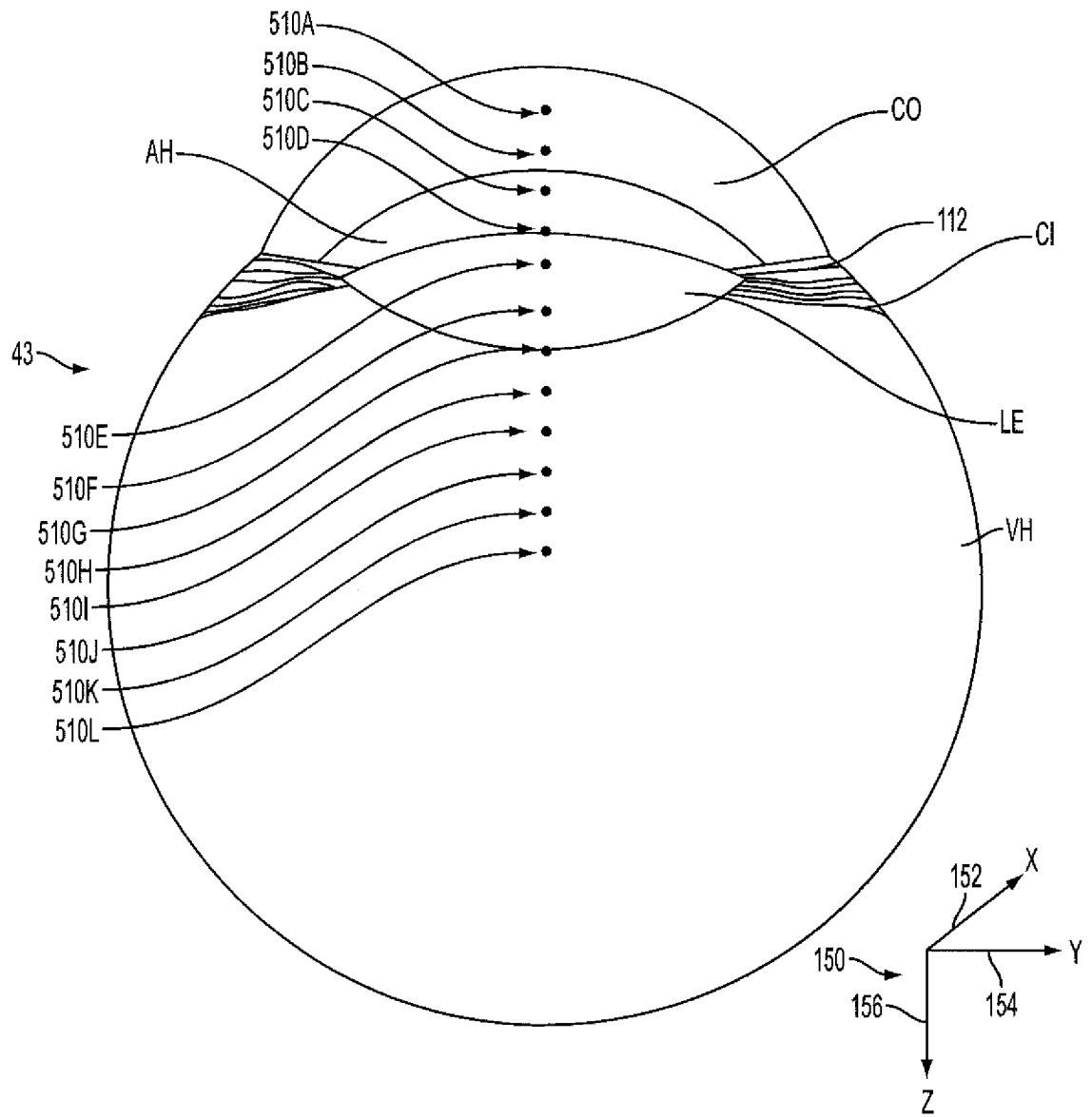
FIG. 5B
