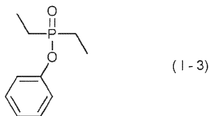
[Chem. 5]
