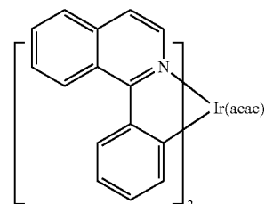
Ir(piq) 2 (acac)
