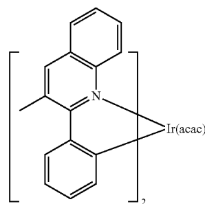
Ir(3-Mepq) 2 (acac)
