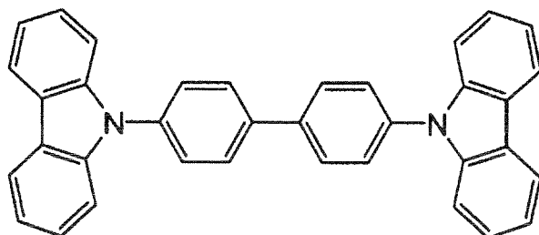
[Chem. 3]
