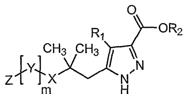
(Ik)
