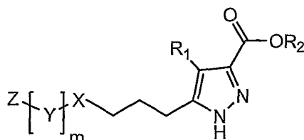
(Ip)
