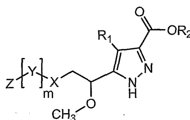
(Io)
