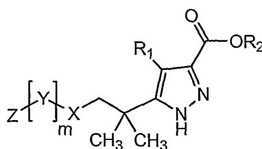
(Im)
