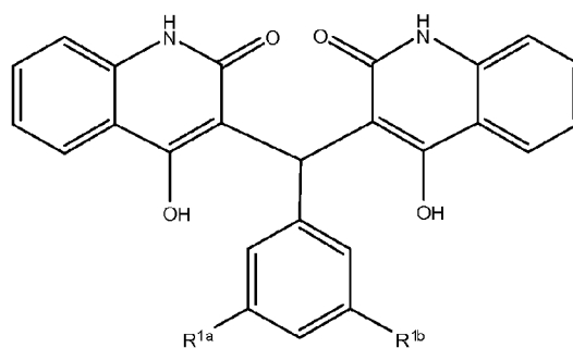
Formula Va
