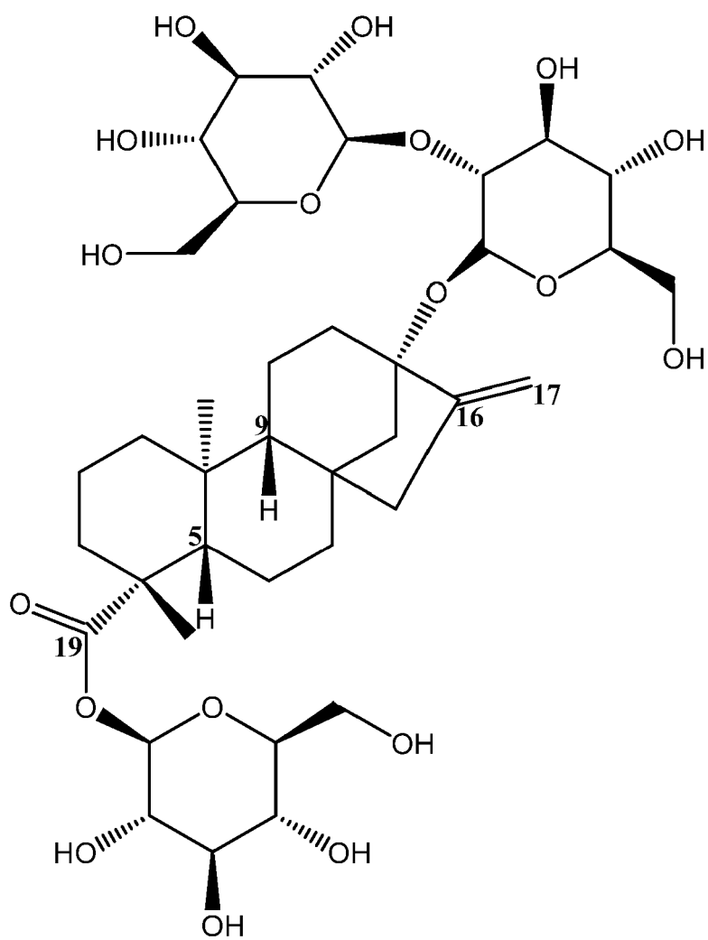
Stevioside
