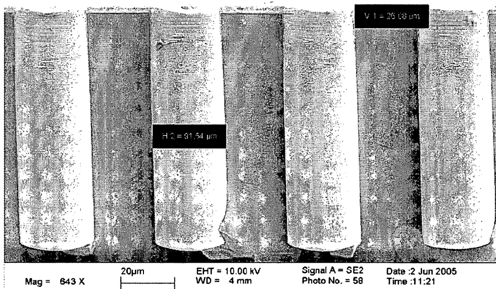
20 um diameter 100um deep filled Via
