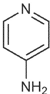
4-aminopyridine
