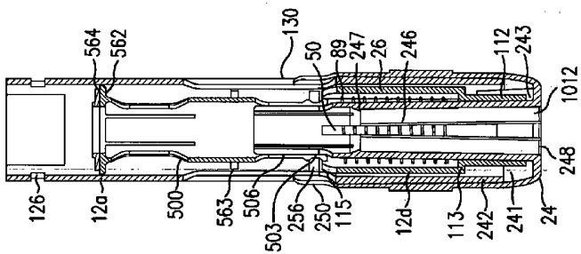
FIG. 18B
