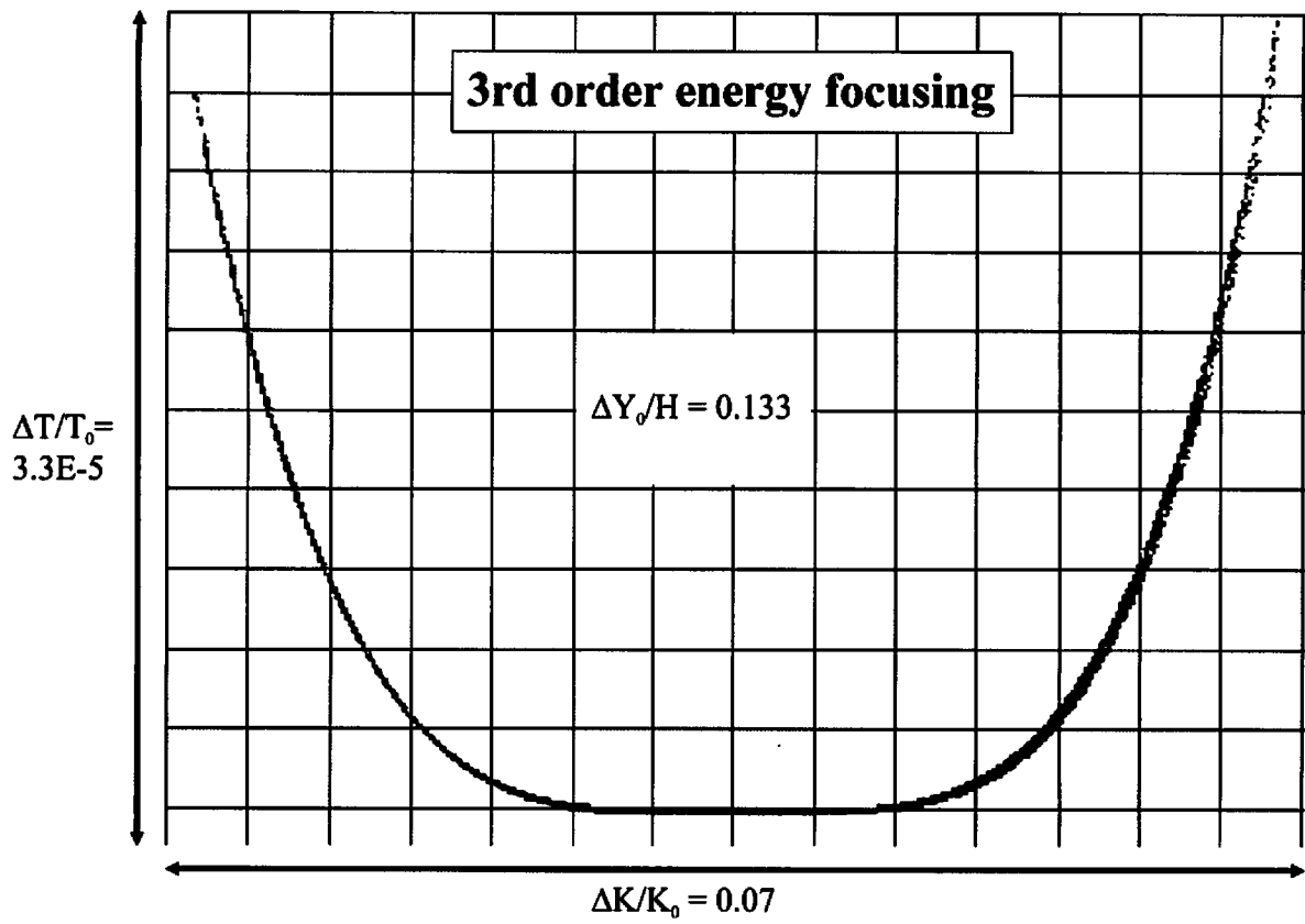
Fig. 5; Prior Art MPA-2-3
