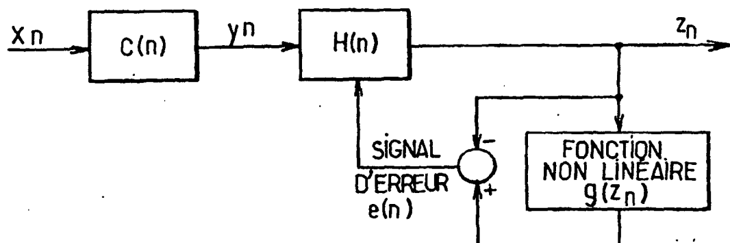
FIG.1a. ÉGALISEUR AUTODIDACTE DE BUSSGANG (ART ANTÉRIEUR)
