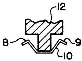
SECTION D-D FIG. 7D
