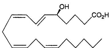
5(S)-HETE
