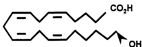
20-HETE
