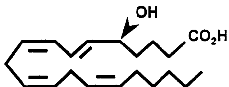
5(S)-HETE
