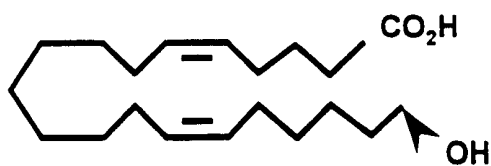
ps 20-HETE
