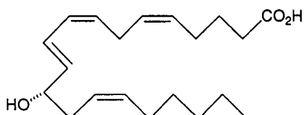
12(S)-HETE
