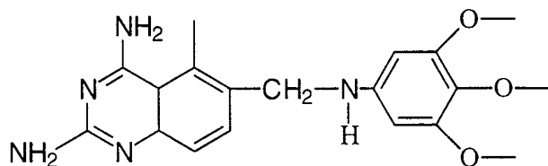
Trimetrexate
