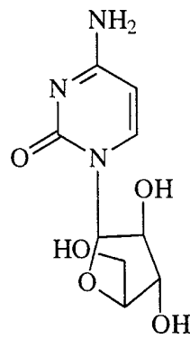
Cytarabine
