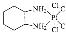
Tetraplatin (Ormaplatin)
