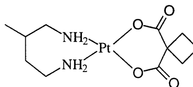
CI-973
