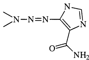
Dacarbazine
