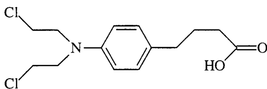
Chlorambucil
