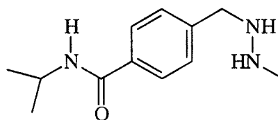
Procarbazine
