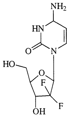
Gemcitabine
