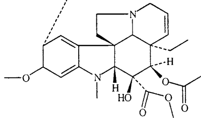
Vinorelbine
