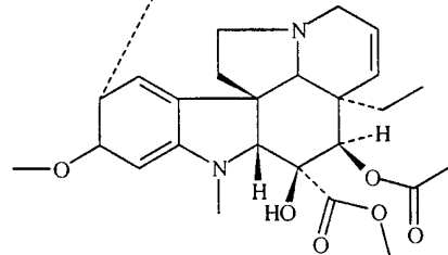
Vinblastine
