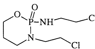
Ifosfamide
