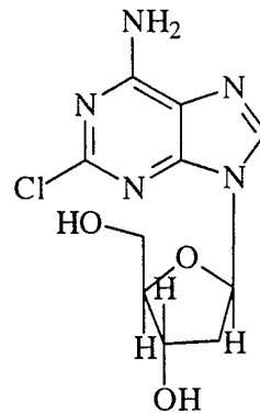
Cladribine
