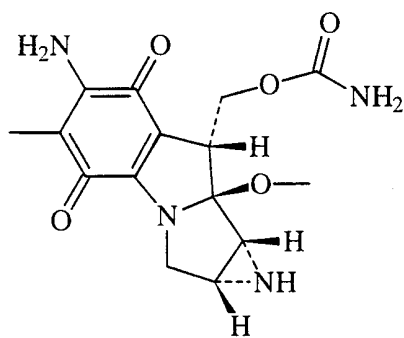
Mitomycin
