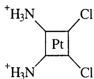
Cisplatin
