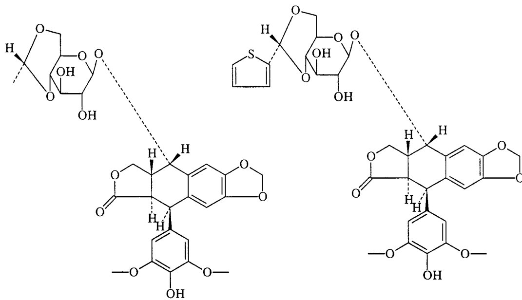
Etoposide
