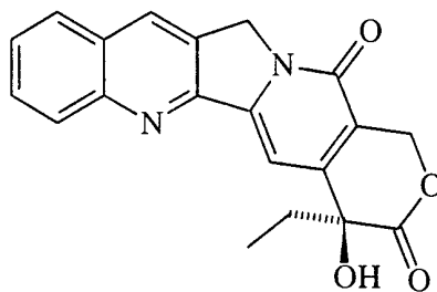
Camptothecin
