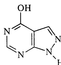
Allopurinol
