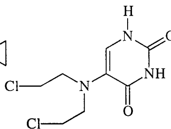
Uracil Mustard
