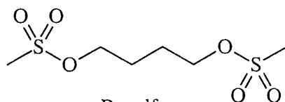
Busulfan
