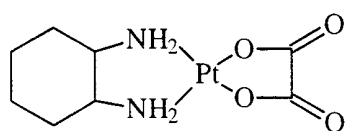
Oxaliplatin
